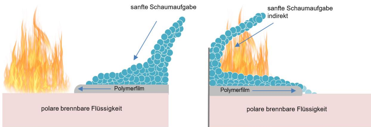
Abb. 1: Löschwirkung von alkoholbeständigem Schaummittel. Ausbildung der Polymersperrschicht zwischen polarem Medium und dem Löschschaum.
