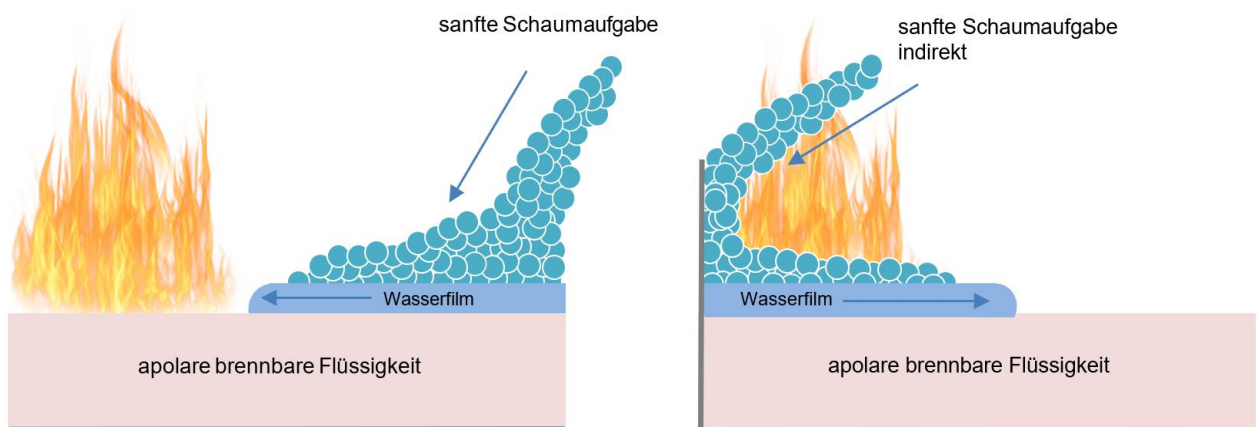
Abb. 2: Löschwirkung wasserfilmbildender Schaummittel (AFFF)
